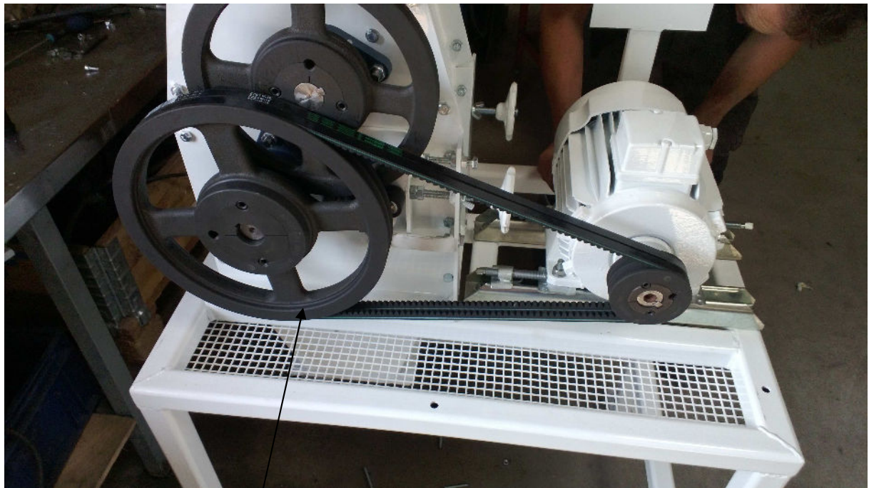
Transmission poules courroies
